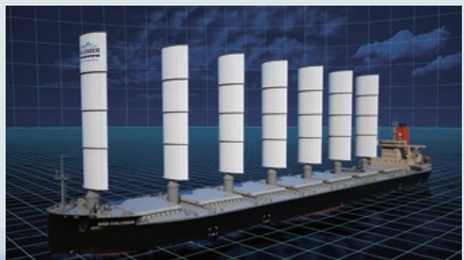
硬翼帆式風力推進装置を搭載した 石炭専用船(2022年運航開始予定)
